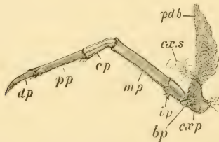
FIG. 78.— Cambarus (Guatemala) penultimate leg. exp , coxopodite; cx.s , coxopoditic setæ; pdbs , podobranchia; bp , basipodite; ip , ischiopodite; mp , meropodite; cp carpopodite; pp , propodite; dp , dactylopodite.
